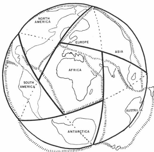
Afbeelding 4. Belangrijke seismotektonische gordels/'plaatgrenzen' (streepjeslijnen) vergeleken met een icosaeëder. 8 (Herdruckt met toestemming van de American Geophysical Union.)
