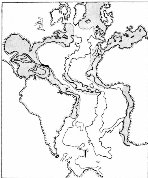
Afbeelding 15. Gebieden (gearceerd) in de Atlantische Oceaan waarvan is vastgesteld dat ze verzonken zijn. 15 (Herdruckt met toestemming van de AAPG.)
