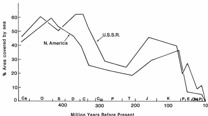
Afbeelding 11. Mate van overstrooming door de zee voor elk fanerozoïsch tijdvak voor de voormalige Sovjetunie en Noord-Amerika. Hoe ouder de geologische periode des te groter de kans dat de mate van overstrooming wordt onderschat omdat de sedimenten zijn geërodeerd of diep begraven liggen onder jongere sedimenten. 7 (Herdruckt met toestemming van Nature .)
