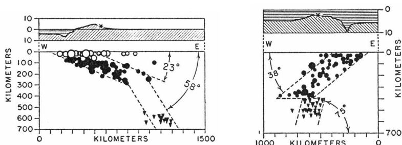
Afbeelding 7. Dwarsdoorsneden door de Peru-Chili-trog (links) en de Bonin-Honshu-boog (rechts), waarop epicentra van aardbevingen te zien zijn. 12 (Herdrukt met toestemming van de Geological Society of America.)
