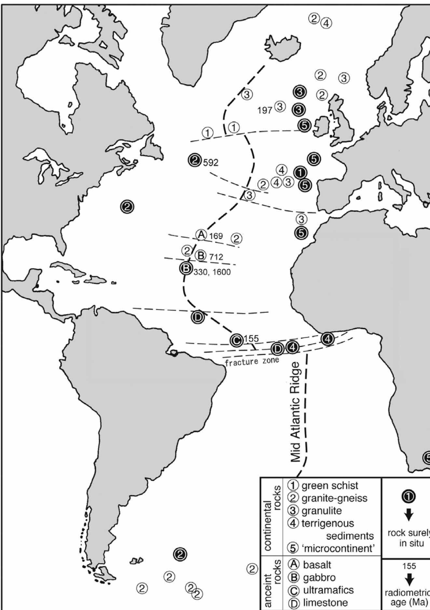
Afbeelding 16. Oude en continentale gesteenten die tot dusver in de Atlantische Oceaan zijn ontdekt (Vasiliev & Yano, 2007).
